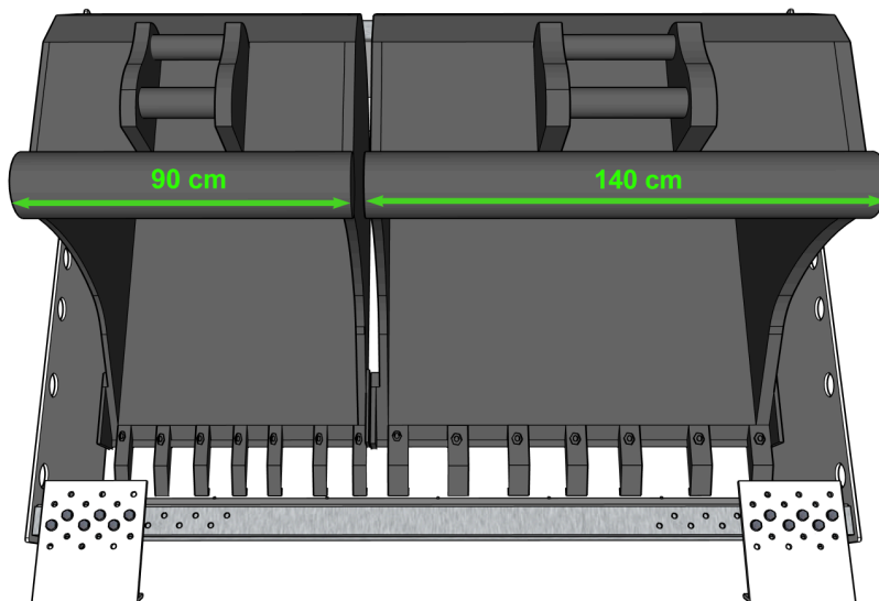
Exemple de configuration de positionnement de godets
